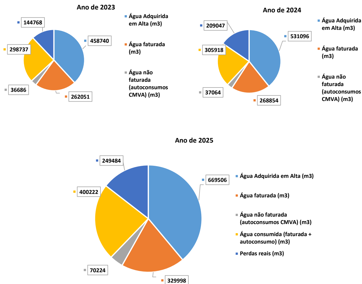
Gráfico 7 - Volume de água adquirida à AgdA, água faturada aos munícipes, autoconsumos, água consumida e perdas reais, no período de 2023 a 2025.
