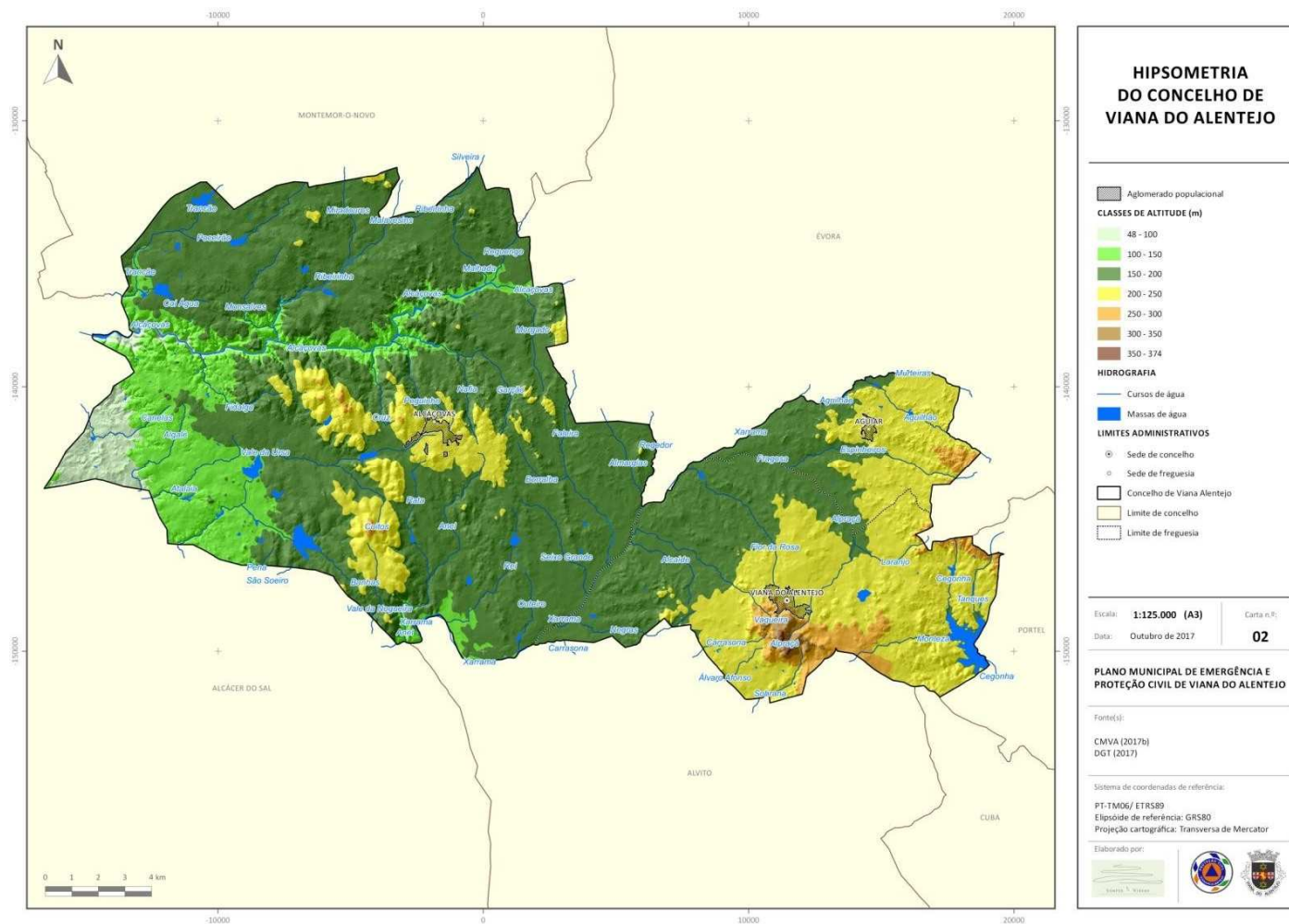
Carta 2. Hipsometria do concelho de Viana do Alentejo
