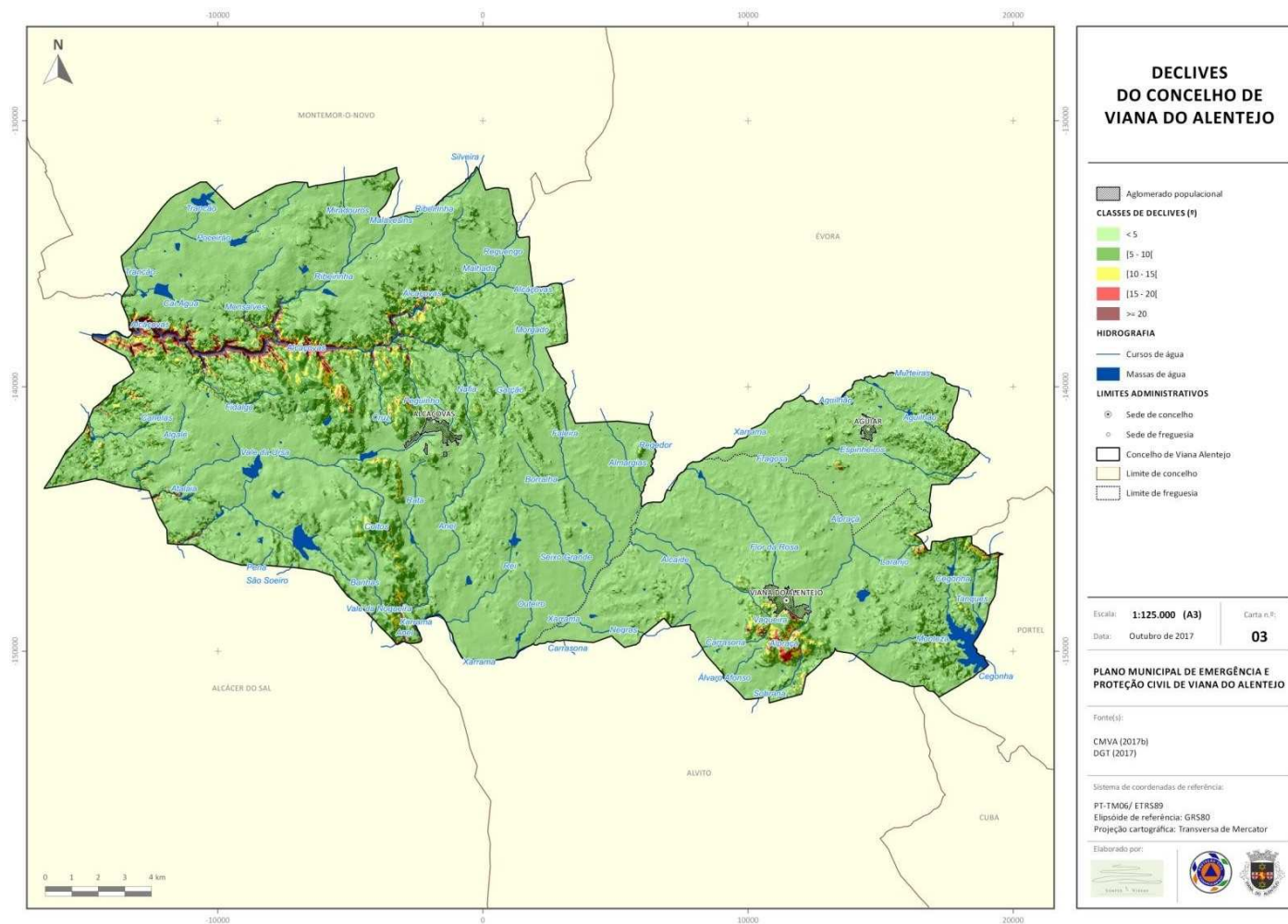
Carta 3. Declives do concelho de Viana do Alentejo
